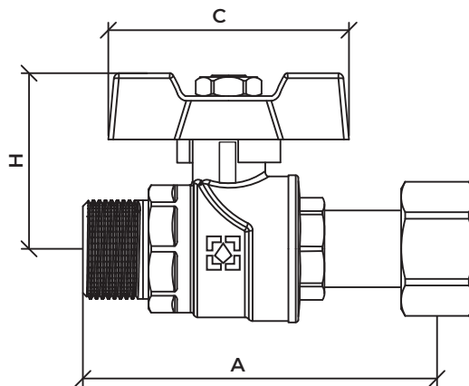
Кран шаровый прямой с накидной гайкой серии Black
