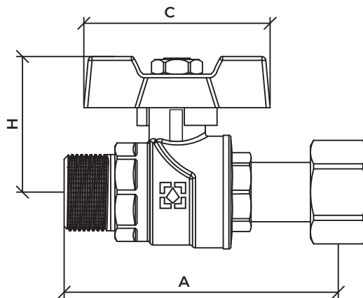
Kulový kohout s převlečnou maticí a vnějším závitem série Black
