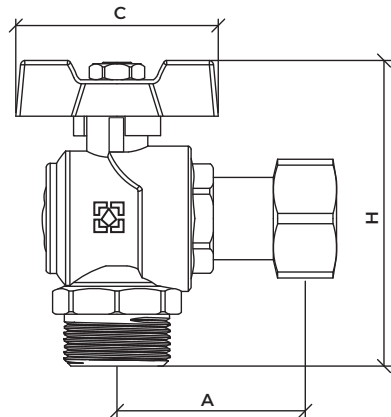
Кран кульовий кутовий з накидною гайкою серії Black
