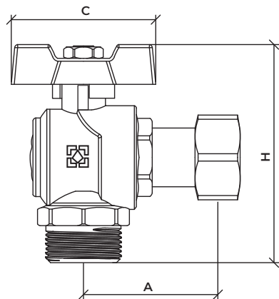
Kulový kohout s převlečnou maticí a vnějším závitem série Black
