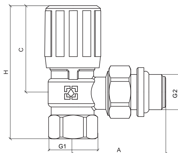
Клапан ручного регулювання ВР-ЗР
