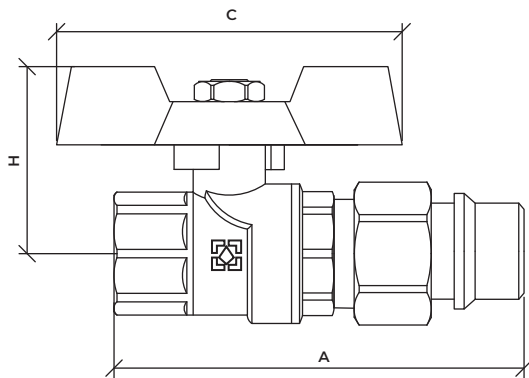
Кран шаровой с разъёмным соединением серия White
