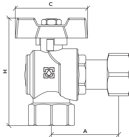
Кран шаровый угловой с накладной гайкой серии Black
