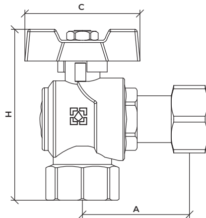
Kulový kohout s převlečnou maticí a vnitřním závitem série Black
