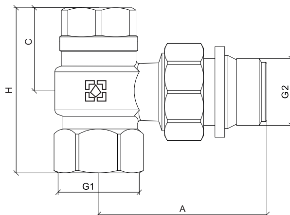
Rohový regulovatelný radiátorový ventil ŠM
