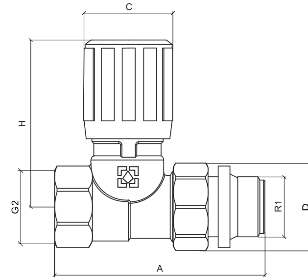
Клапан радіаторний ручного регулювання прямий ВР-ЗР
