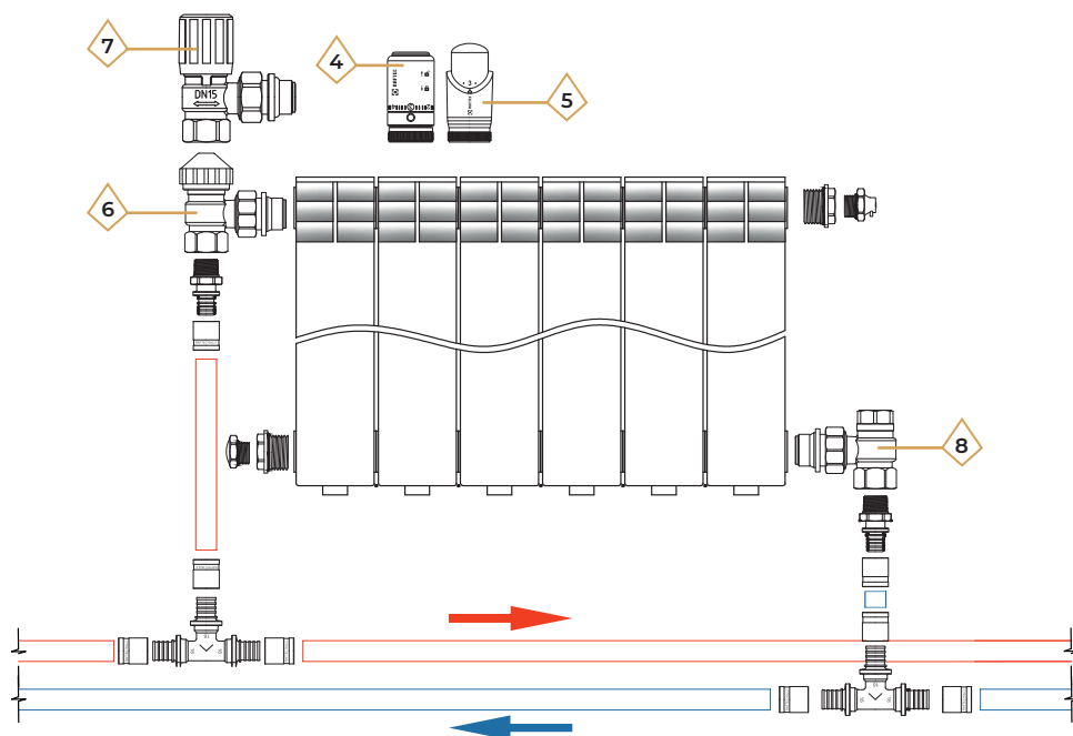
Схема бокового підключення радіатора з кутовими кранами
