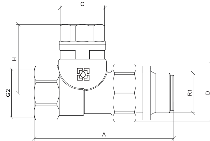
Кран настроювальний прямий ВР-ЗР
