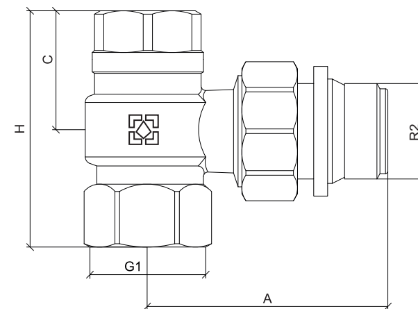
Кран настроювальний кутовий ВР-ЗР
