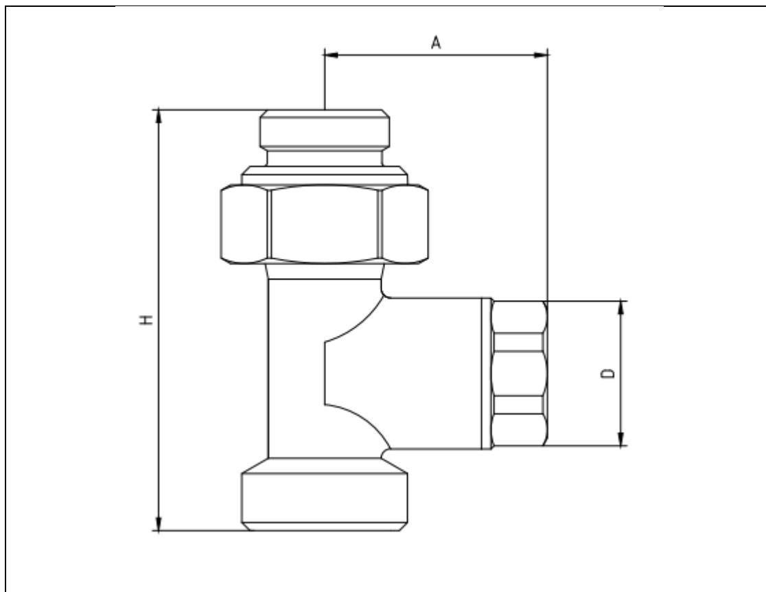
Spodní přípojovací jednotka radiátoru – Přímá
