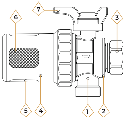
Magnetický filtr RMGHB02
