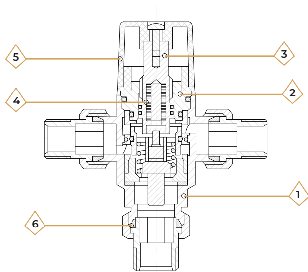
Termostatický třícestný směšovací ventil
